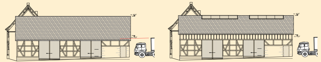
Der Bestand der Querscheune (links) und die Planung mit aufgestockten ersten Geschoss (rechts)
